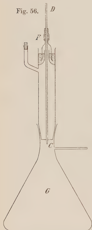
Aus „Moser, Die Reindarstellung von Gasen“.
