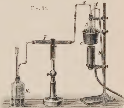
Aus Muspratts Chemie, 4. Aufl., Bd. VII.
