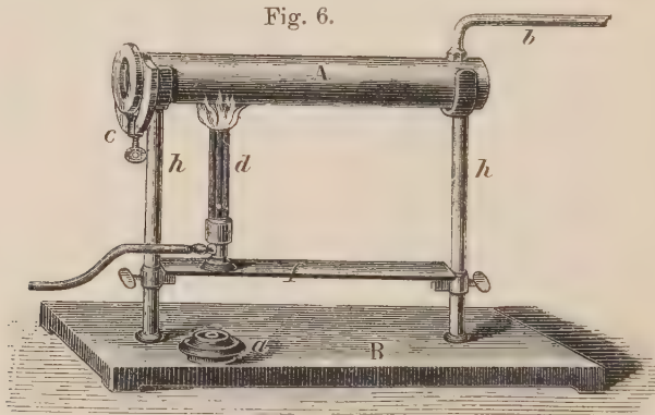
Aus Bender, Anleit. z. Darst. anorg. chem. Präp.
