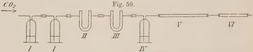
Stabflaschenkohlenäure. Angenommene Verunreinigungen: Sauerstoff, Kohlendioxyd, Schwefelwasserstoff. I. Chromazetat oder Titantrichlorid. II. Kaliumbikarbonat in kleinen Stücken. III. Kupfervitriolbimsstein. IV. Konz. Schwefelsäure. V. Kupferasbest, erhitzt auf etwa 700°. VI. Kupferoxydasbest, auf etwa 700–800°.
