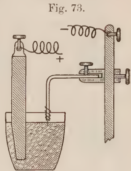
Fig. 73. Aus Ber. d. d. chem. Ges. 35 (1902).
