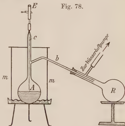
Aus Ostwald-Luther S. 636.
